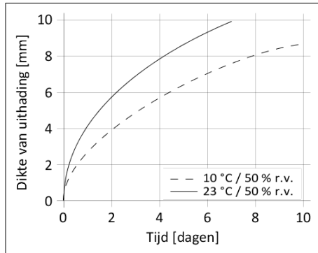
Figuur 1: Uithardingsnelheid SikaTack®-DRIVE (60min)
