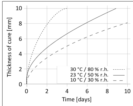
Diagram 1: Uithardingsssnelheid Sikaflex®-668
