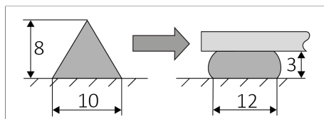
Figuur 1: Aanbevolen rupsconfiguratie
