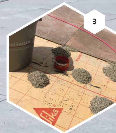
3 SCHÖNOX EP DRAIN gemischt mit SCHÖNOX MONOKORN in Batzenform auf den Boden aufbringen.*
