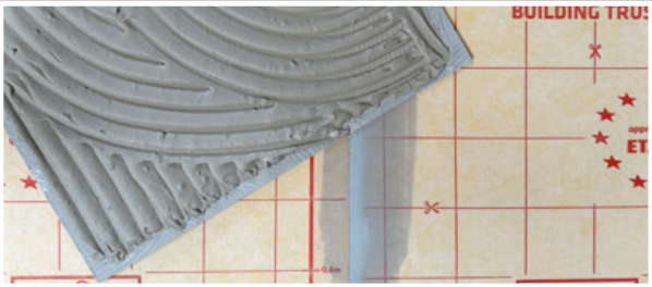
Verlegung von keramischen Belägen / verfärbungsfreiem Naturstein im Battering-Verfahren
