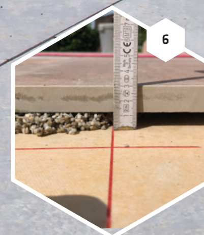
6 Bei Abschlüssen die Plattenränder mit SCHÖNOX EP DRAIN unterfütern.
