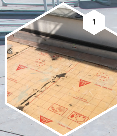
1 Abdichtung mit dem Dichtkleber SCHÖNOX iFIX® und der Abdichtungsbahn SCHÖNOX AB 30/ AB 10.
