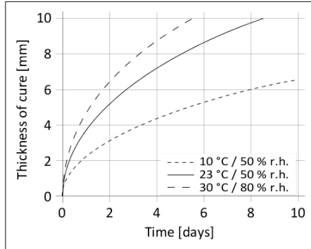
Schema 1: Uithardingsssnelheid Sikaflex®-254
