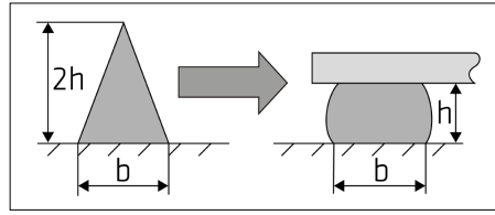
Afbeelding 1: Aanbevolen rupsvorm
