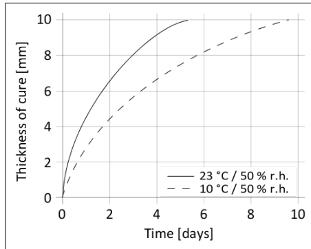
Figuur 1: Doorhardingsnelheid Sikaflex®-228
