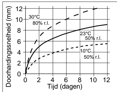
Schema 1: Uithardingsnelheid voor Sikaflex®260 N
